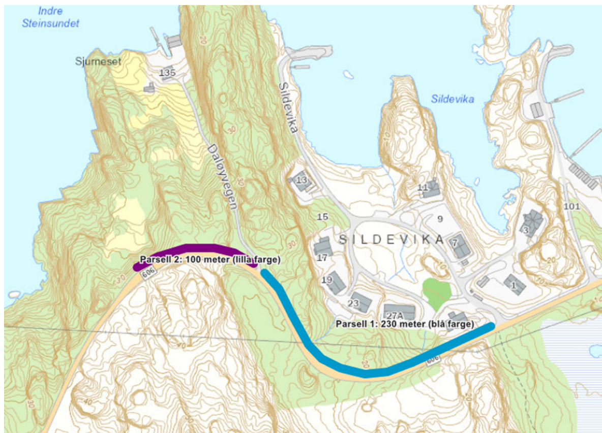
Figur 1: Situasjonsplan som viser strekke aktuell for samfinansiering.
